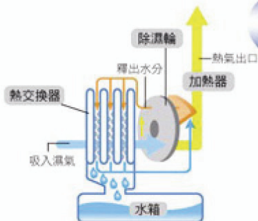
除濕輪運轉圖
